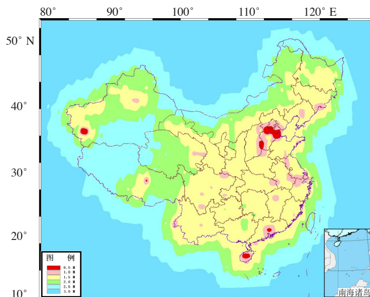
图1 中国地震台网现有地震监测能力分布图
