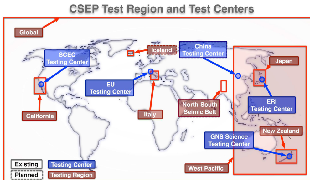
图9 国际地震可预测性合作研究（CSEP）计划的全球测试区（红色矩形）和检验中心（蓝色圆圈）的分布图（引自美国南加州地震中心主任T. Jordan报告）
