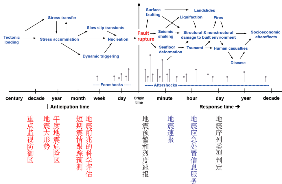
图2 地震监测预报的主要科技问题和主要科技产品 (底图基于美国南加州地震中心主任T. Jordan报告修改)
