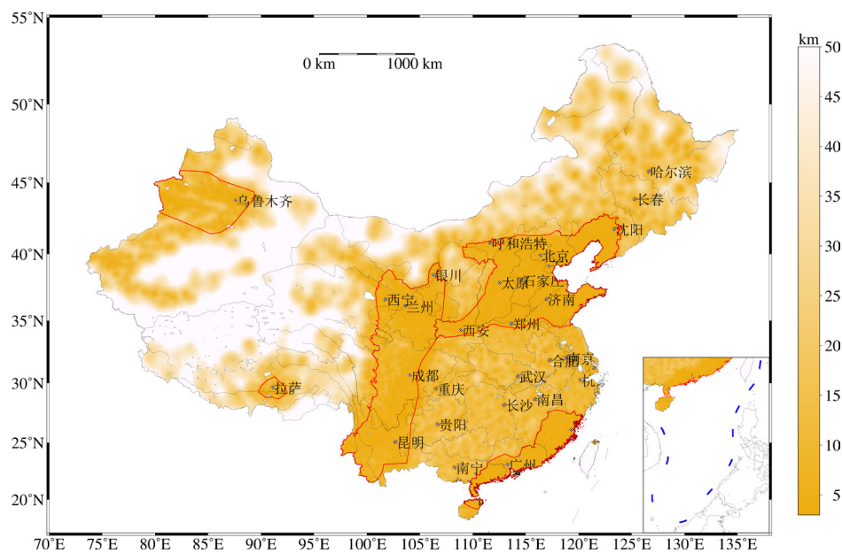
图6 2020年中国大陆地震烈度速报能力分布
